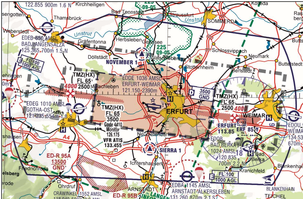
Darstellung der IFR-Endanflüge am Beispiel Erfurt
