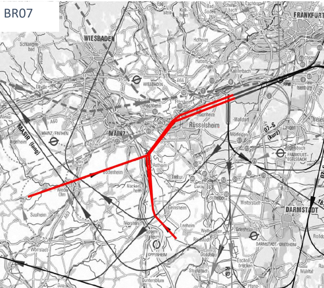
Segmentierter Anflug bei Betriebsrichtung 07 (Ostwind)
